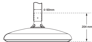
Pendant Mounted
